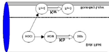
Gambar 1 Zone Reaksi dalam pipa Sumber : EPANET User Manual
