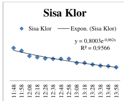
Gambar 1. Hasil Eksponensial Peluruhan Klor Sumber : Hasil Penelitian
