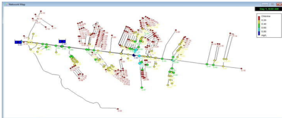
Gambar 5. Hasil Simulasi 1 Sebaran Sisa Klor Pada Pukul 08.00
