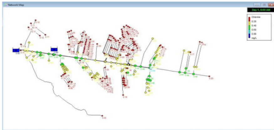
Gambar 6. Hasil Simulasi 2 pada pukul 08.00
