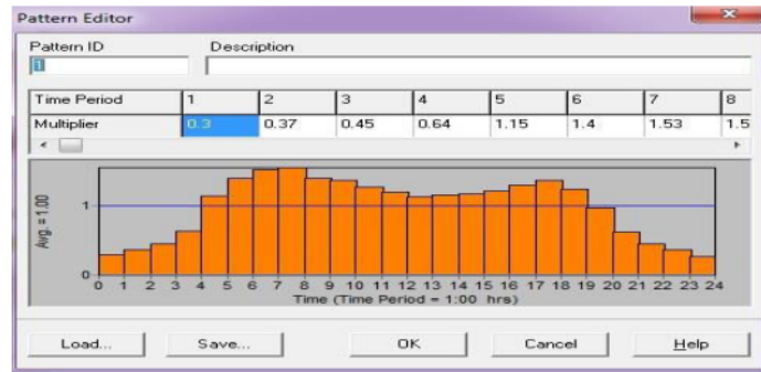
Gambar 3. Pettern selama 24 jam
