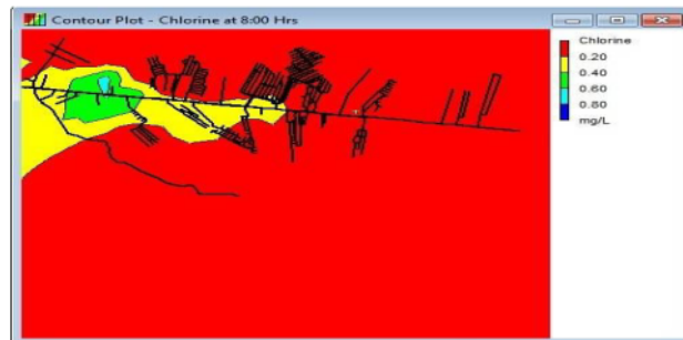
Gambar 4. Contour Plot Sebaran Klor pada 08.00
