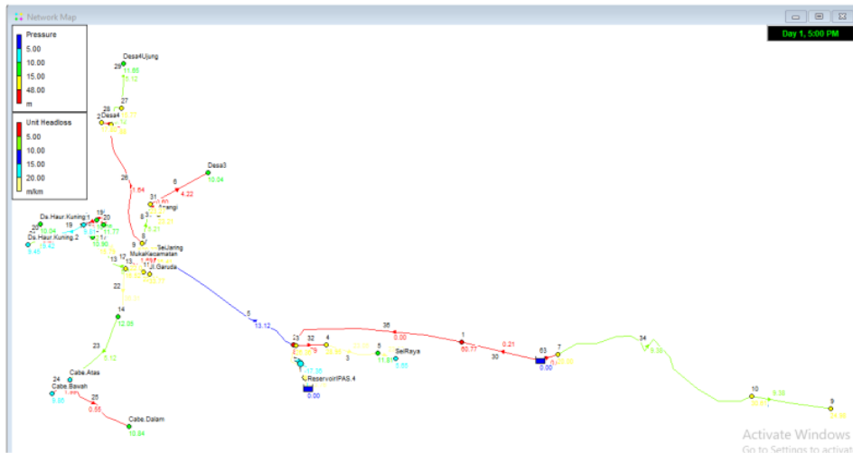
Gambar 3.9 Hasil Simulasi Peningkatan Kinerja Dengan Mengganti Dua Buah Pompa
