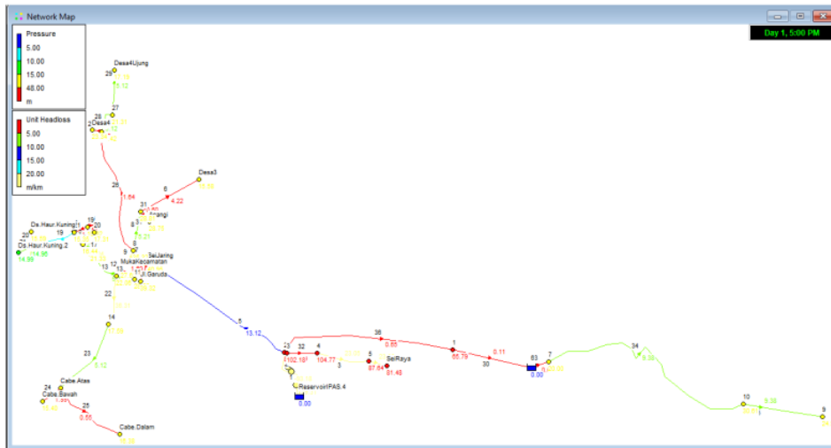
Gambar 3.15 Hasil Simulasi Peningkatan Kinerja
