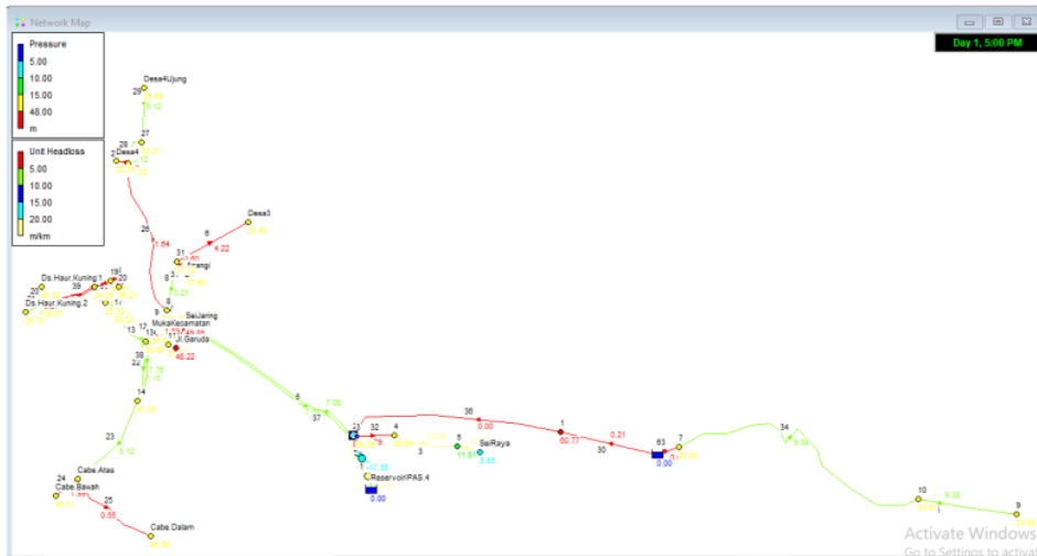
Gambar 3.12 Hasil Simulasi Peningkatan Kinerja Dengan Memperbesar Diameter
