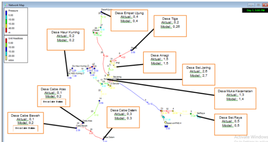
Gambar 3.3 Hasil Kegiatan Validasi Model Jaringan
