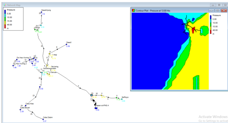
Gambar 3.5 Lokasi Sisa Tekanan Yang Belum Memenuhi Standar
