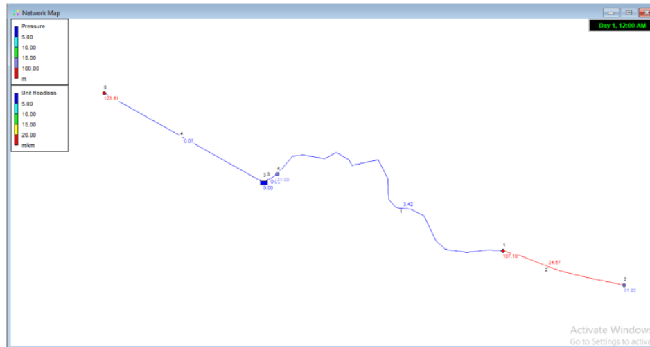
Gambar 3.18 Hasil Simulasi Model IPA Sambung Makmur
