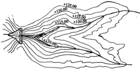
Gambar 1. Lay out dari waduk
