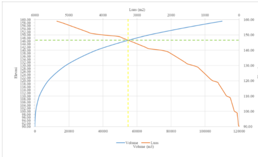
Gambar 5. Grafik Lengkung Kapasitas Waduk
