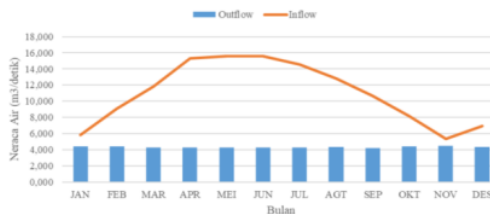
Gambar 7. Grafik Neraca Air di Waduk Tapin
