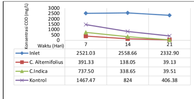
Gambar 2. Grafik Konsentrasi COD pada effluent LBB-AHBP
