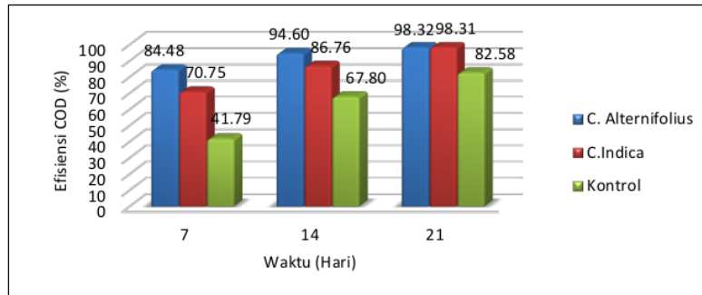
Gambar 3. Grafik Efisiensi COD pada Sistem LBB-AHBP
