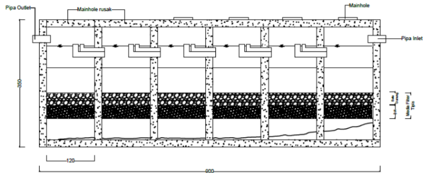
Gambar 2 Layout IPAL Komunal setelah 6 tahun
