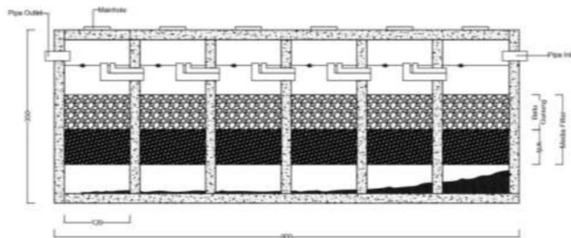
Gambar Layout IPAL Komunal awal pembangunan
