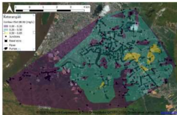
Gambar 10. Contour Plot simulasi 3 pada 08:00
