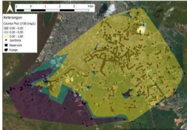
Gambar 5. Contour plot sebaran klor pada 17:00
