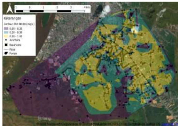
Gambar 8. Contour Plot simulasi 2 pada 08:00
