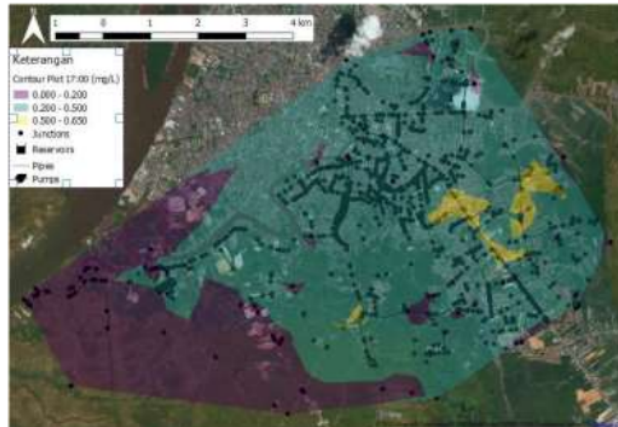
Gambar 11. Contour Plot simulasi 3 pada 17:00
