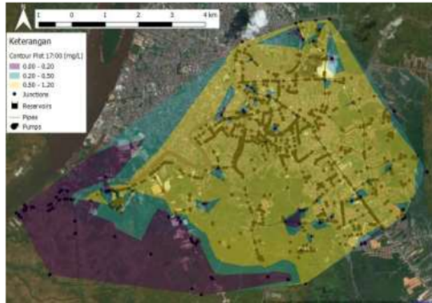
Gambar 7. Contour Plot simulasi 1 pada 17:00
