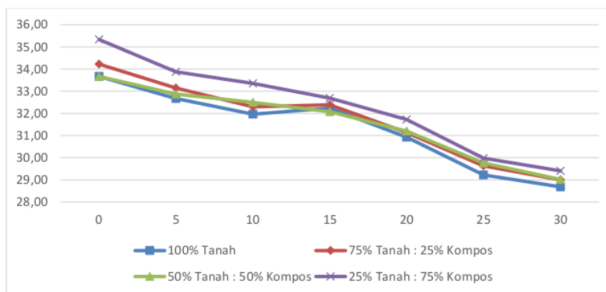
Gambar 1. Grafik Perubahan Suhu Rata-rata per 5 Hari
