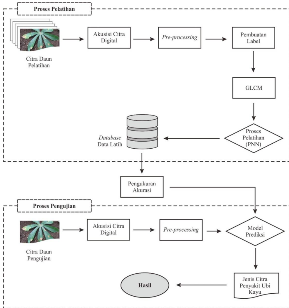
Gambar 2. Alur Sistem
