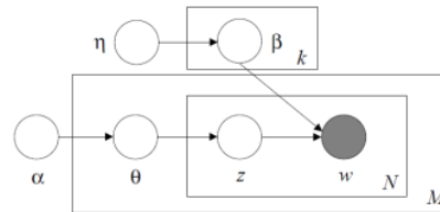
Gambar 6. Representasi model probabilistik LDA yang dihaluskan
