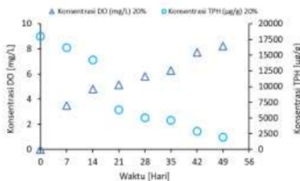
Gambar 5. Pengaruh Konsentrasi Oksigen dan terhadap Reduksi TPH ( activated sludge 15%(v/v))
