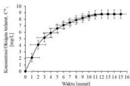
Gambar 3. Hubungan antara konsentrasi oksigen terlarut terhadap waktu
