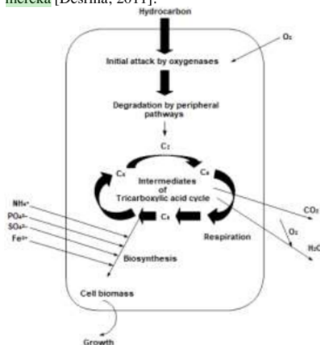
Gambar 1. Prinsip utama degradasi aerobik hidrokarbon oleh mikroorganisme
