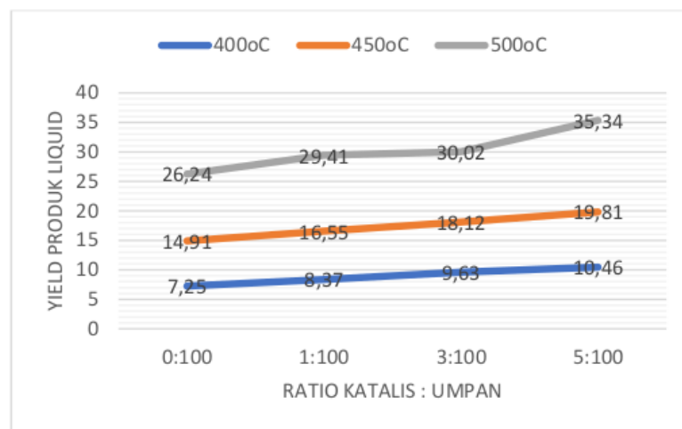
Gambar 3 Pengaruh rasio katalis terhadap yield produk liquid hasil pirolisis ban bekas pada berbagai temperature.
