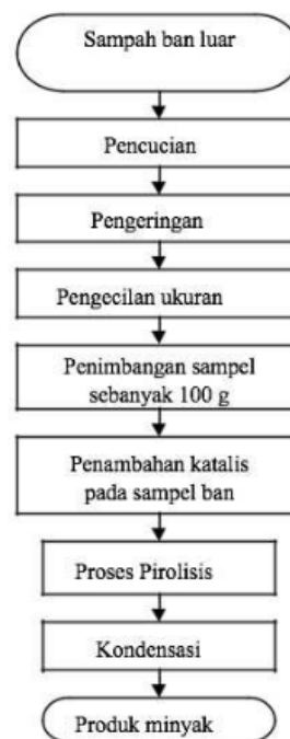
Gambar 2. Diagram alir proses pirolisis.
