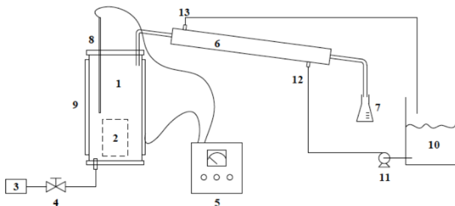
Gambar 1. Rangkaian alat pirolisis ban bekas
