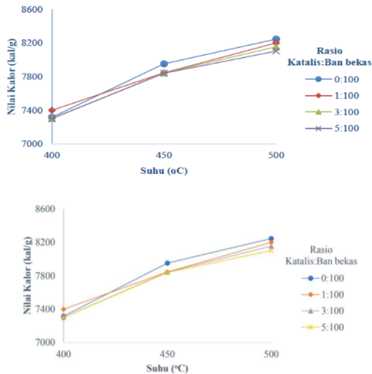
Gambar 4. Pengaruh temperatur dan rasio penambahan katalis terhadap nilai kalor fuel dari pirolisis ban luar bekas.
