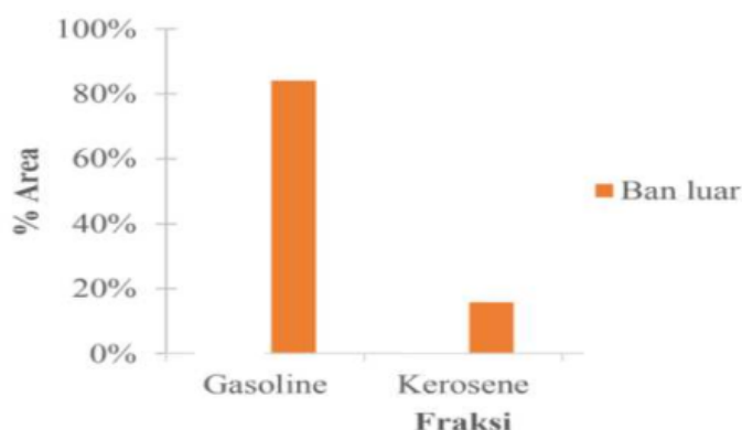
Gambar 5. Fraksi bahan bakar dalam produk liquid hasil pirolisis ban luar
