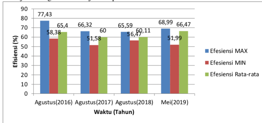
Gambar 8. Grafik Kinerja Efisiensi Cooling Tower
