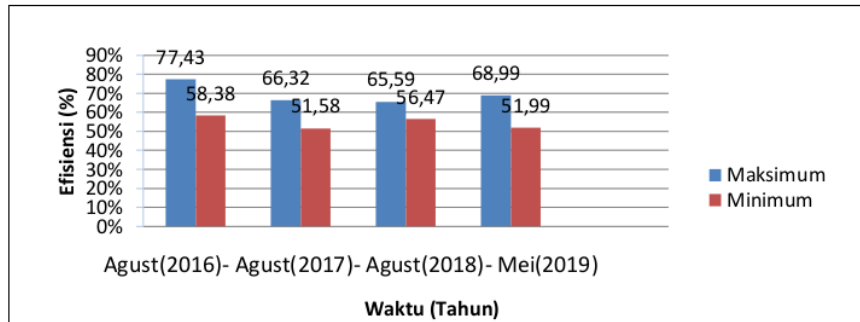
Gambar 5. Grafik Efisiensi Cooling Tower
