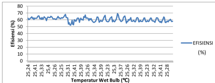
Gambar 4. Grafik Efisiensi Cooling Tower
