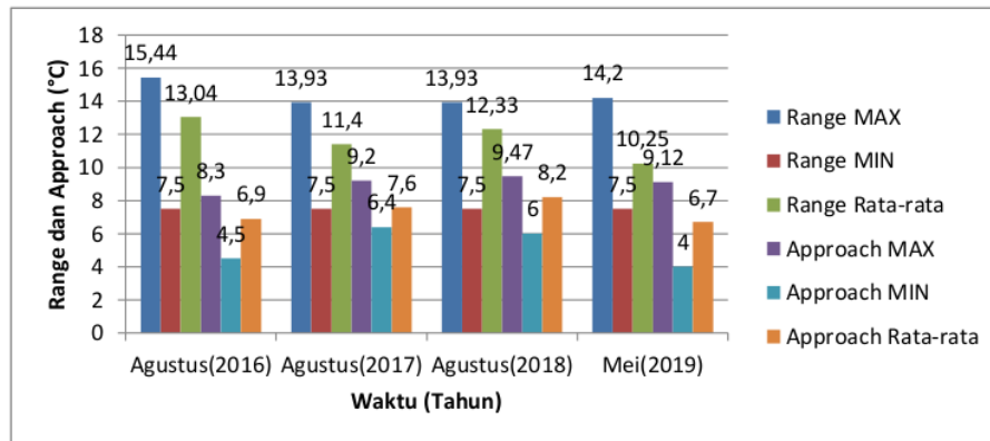
Gambar 9. Grafik Kinerja Range dan Approach Cooling Tower
