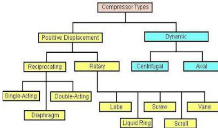
Gambar 1. Jenis-Jenis Kompresor
