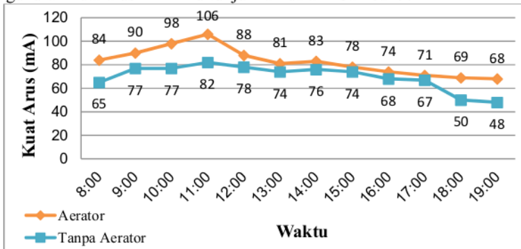
Gambar 9. Grafik Perbandingan Kuat Arus Zn+Zn
