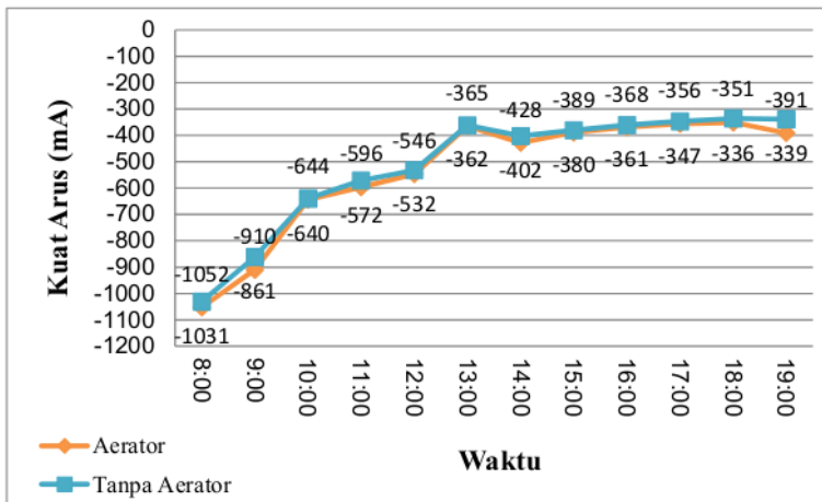
Gambar 10. Grafik Perbandingan Kuat Arus Cu+Zn
