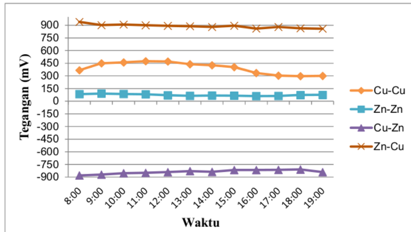
Gambar 19. Grafik Perbandingan Tegangan Tanpa Menggunakan Aerator
