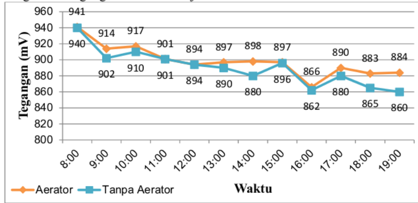
Gambar 15. Grafik Perbandingan Tegangan Zn+Cu
