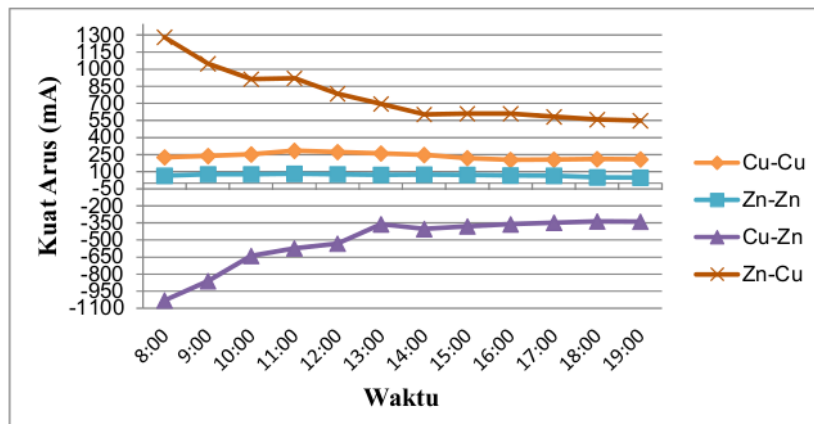
Gambar 17. Grafik Perbandingan Kuat Arus Tanpa Menggunakan Aerator
