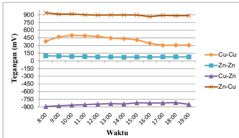
Gambar 18. Grafik Perbandingan Tegangan Menggunakan Aerator
