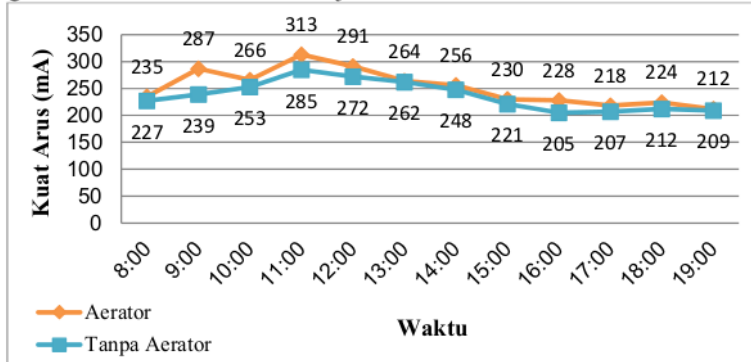
Gambar 8. Grafik Perbandingan Kuat Arus Cu+Cu
