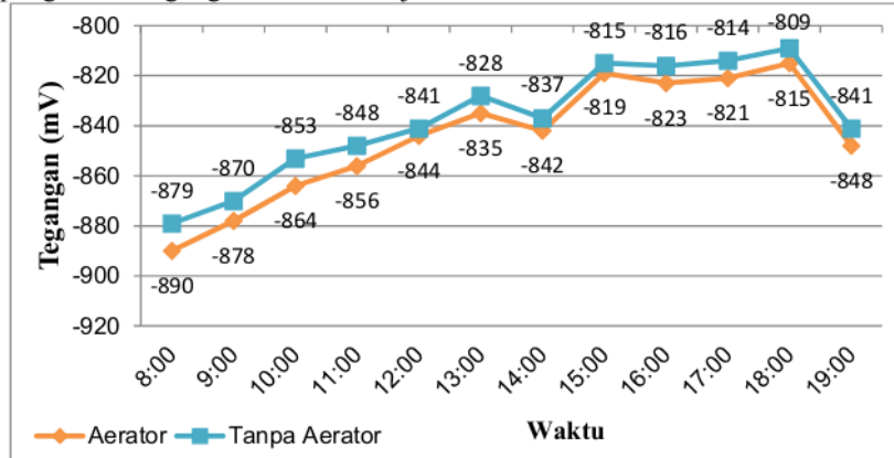
Gambar 14. Grafik Perbandingan Tegangan Cu+Zn
