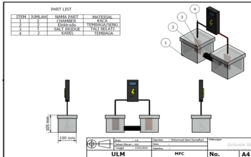
Gambar 6. Desain MFC
