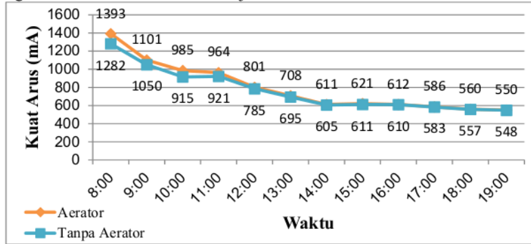
Gambar 11. Grafik Perbandingan Kuat Arus Zn+Cu
