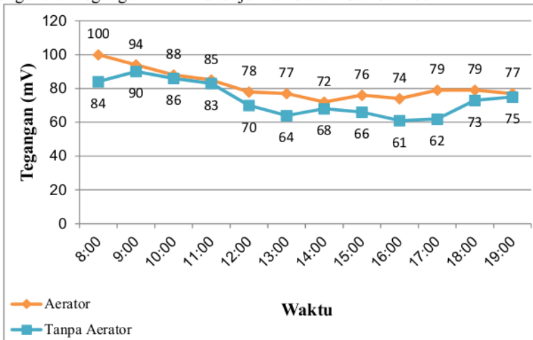
Gambar 13. Grafik Perbandingan Tegangan Zn+Zn
