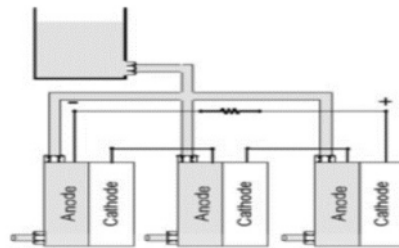
Gambar 3. Skema Stack
