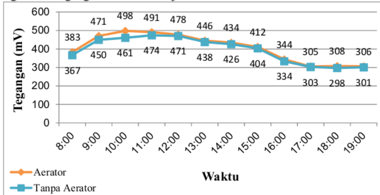
Gambar 12. Grafik Perbandingan Tegangan Cu+Cu
