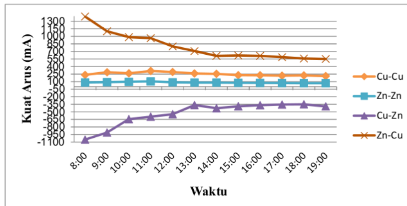
Gambar 16. Grafik Perbandingan Kuat Arus Menggunakan Aerator
