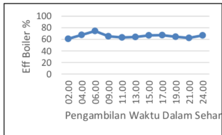
Gambar 12. Effisiensi Boiler Unit 2 Tanggal 17 Agustus 2017
