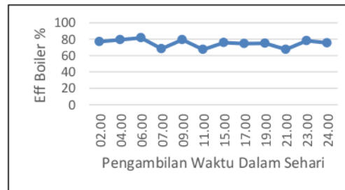
Gambar 20. Efisiensi Boiler Unit 4 Tanggal 14 Agustus 2017
