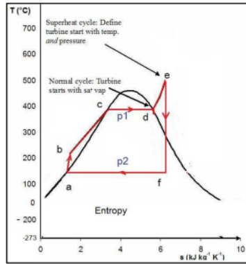
Gambar 1. Diagram T-s Siklus PLTU (Siklus Rankine)
