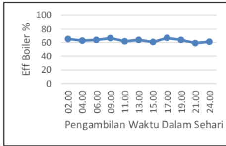
Gambar 11. Effisiensi Boiler Unit 2 Tanggal 16 Agustus 2017
