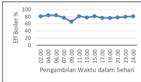
Gambar 16. Efisiensi Boiler Unit 4 Tanggal 10 Agustus 2017
