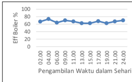
Gambar 5. Efisiensi Boiler Unit 2 Tanggal 10 Agustus 2017
