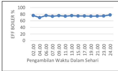
Gambar 14. Efisiensi Boiler Unit 4 Tanggal 8 Agustus 2017
