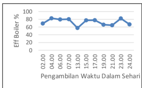
Gambar 23. Effisiensi Boiler Unit 4 Tanggal 17 Agustus 2017
