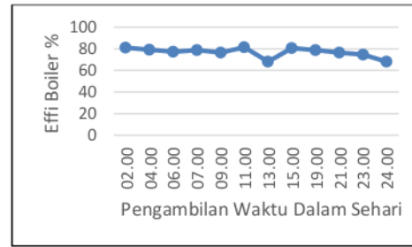
Gambar 18. Efisiensi Boiler Unit 4 Tanggal 12 Agustus 2017
