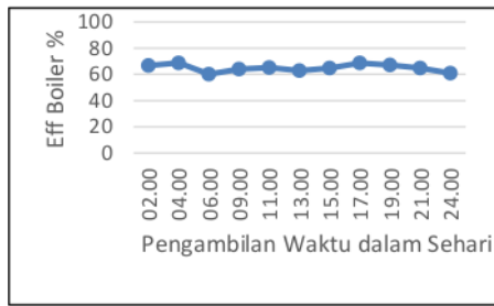
Gambar 3. Efisiensi Boiler Unit 2 Tanggal 8 Agustus 2017
