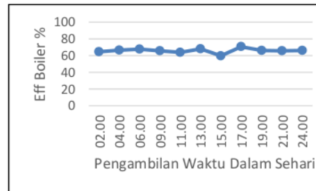
Gambar 10. Efisiensi Boiler Unit 2 Tanggal 15 Agustus 2017
