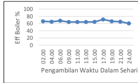
Gambar 9. Efisiensi Boiler Unit 2 Tanggal 14 Agustus 2017
