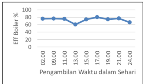
Gambar 15. Efisiensi Boiler Unit 4 Tanggal 9 Agustus 2017
