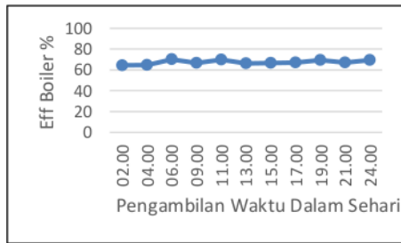
Gambar 4. Efisiensi Boiler Unit 2 Tanggal 9 Agustus 2017
