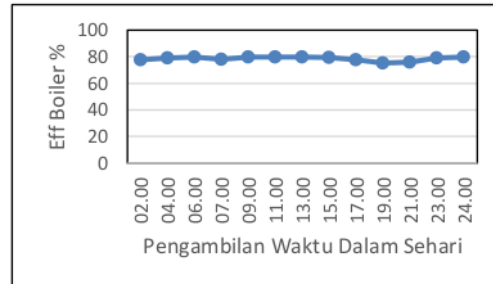
Gambar 19. Efisiensi Boiler Unit 4 Tanggal 13 Agustus 2017
