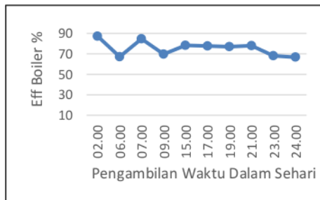
Gambar 17. Efisiensi Boiler Unit 4 Tanggal 11 Agustus 2017
