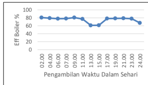
Gambar 21. Efisiensi Boiler Unit 4 Tanggal 15 Agustus 2017
