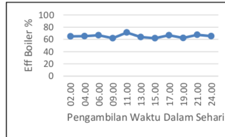
Gambar 8. Efisiensi Boiler Unit 2 Tanggal 13 Agustus 2017
