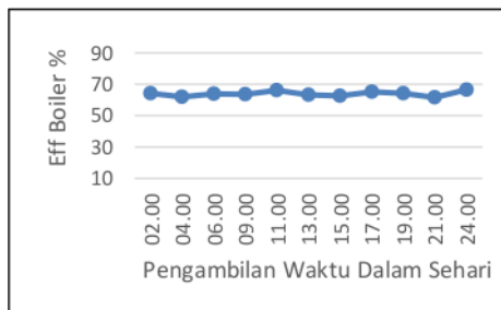
Gambar 6. Efisiensi Boiler Unit 2 Tanggal 11 Agustus 2017
