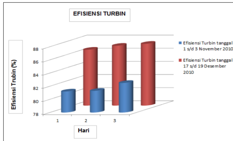
Gambar 10. Efisiensi Turbin
