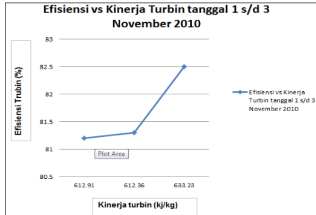
Gambar 11. Grafik Kinerja vs Efisiensi Sebelum Perbaikan Tanggal 1 November s/d 3 November 2010
