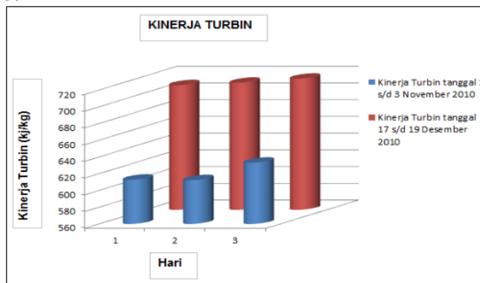
Gambar 9. Kinerja Turbin
