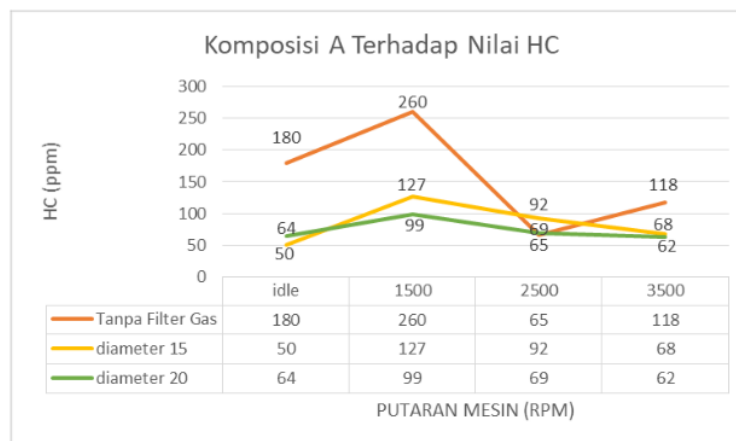
Gambar 9. Komposisi A Terhadap Nilai HC
