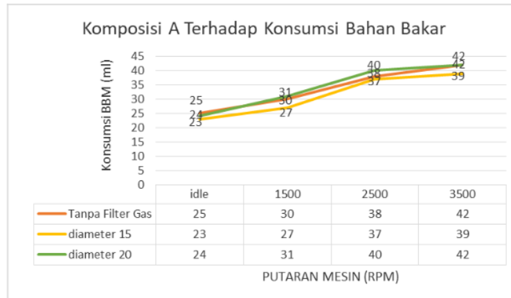
Gambar 13. Komposisi A Terhadap Konsumsi Bahan Bakar
