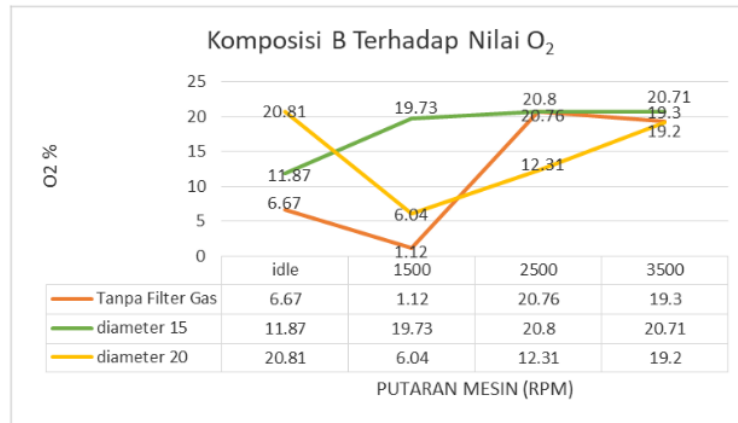
Gambar 12. Komposisi B Terhadap Nilai O 2
