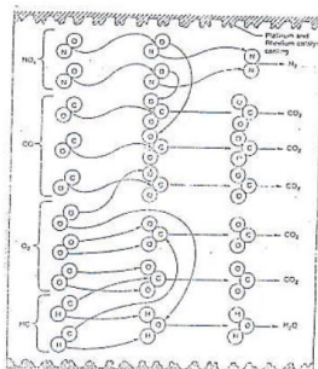
Gambar 1. Perubahan Reaksi Kimia
