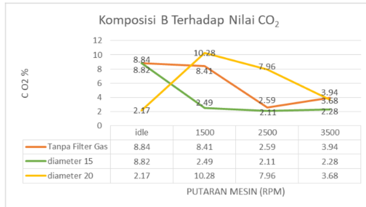
Gambar 6. Komposisi B Terhadap Nilai CO 2
