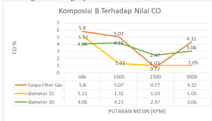
Gambar 8. Komposisi B Terhadap Nilai CO
