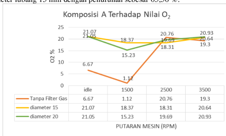
Gambar 11. Komposisi A Terhadap Nilai O 2
