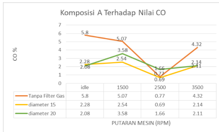
Gambar 7. Komposisi A Terhadap Nilai CO
