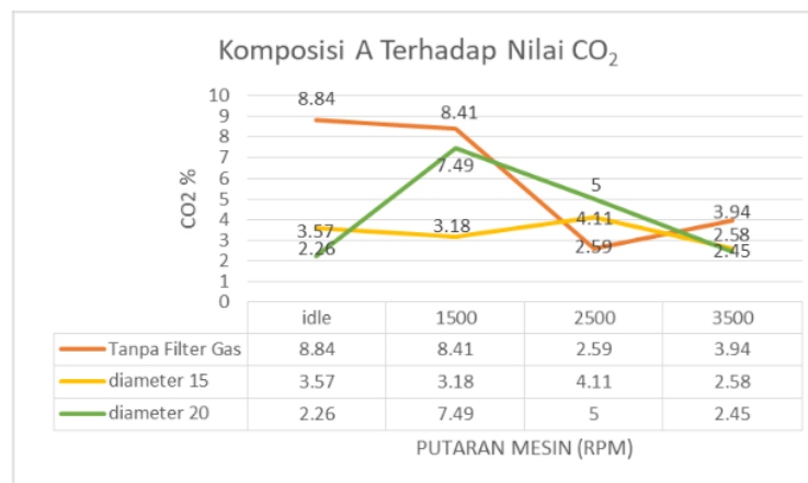
Gambar 5. Komposisi A Terhadap Nilai CO 2
