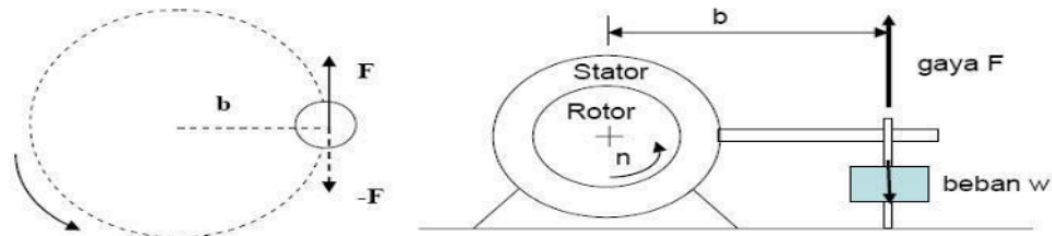
Gambar 2. Torsi Pada Motor
