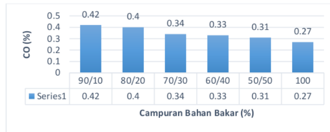
Gambar 11. Grafik Perbandingan Emisi CO
