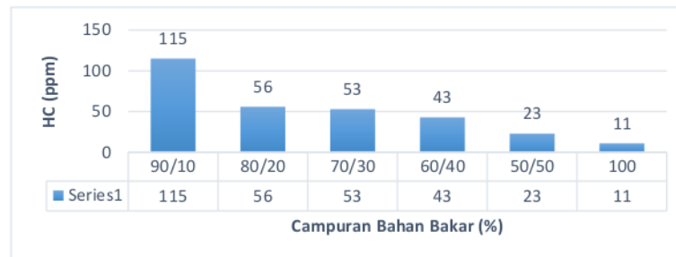
Gambar 10. Grafik Perbandingan Emisi HC
