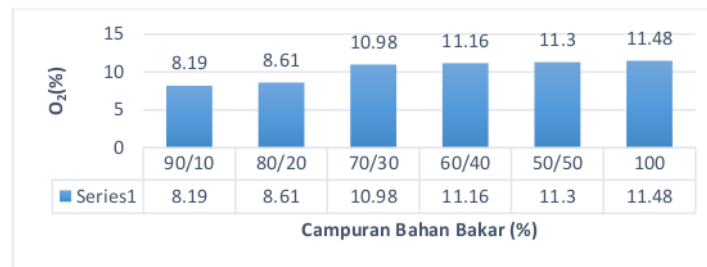
Gambar 13. Grafik Perbandingan Emisi O 2
