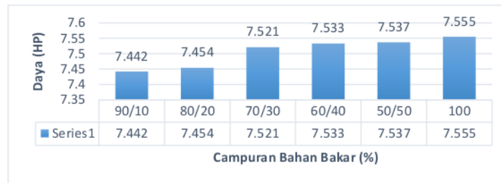
Gambar 8. Grafik Perbandingan Daya Mesin
