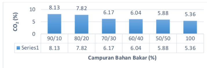
Gambar 12. Grafik Perbandingan Emisi CO 2
