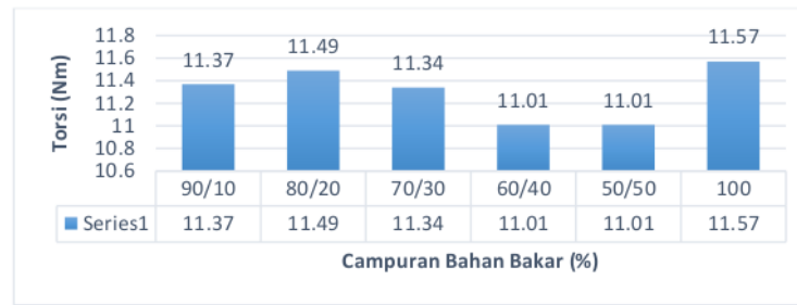
Gambar 9. Grafik Perbandingan Torsi Mesin
