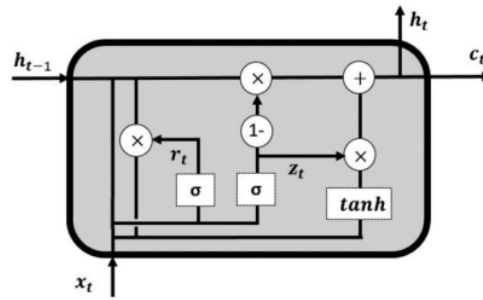
Fig. 5. GRU Architecture
