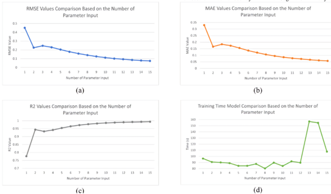
Fig. 9. Model Performance (a) RMSE Values, (b) MAE Values, (c) R2 Values, (d) Training Time
