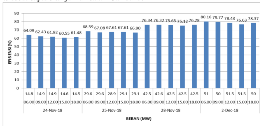
Gambar 7. Grafik Efisiensi Cooling Tower pada Beban dan Waktu Tertentu
