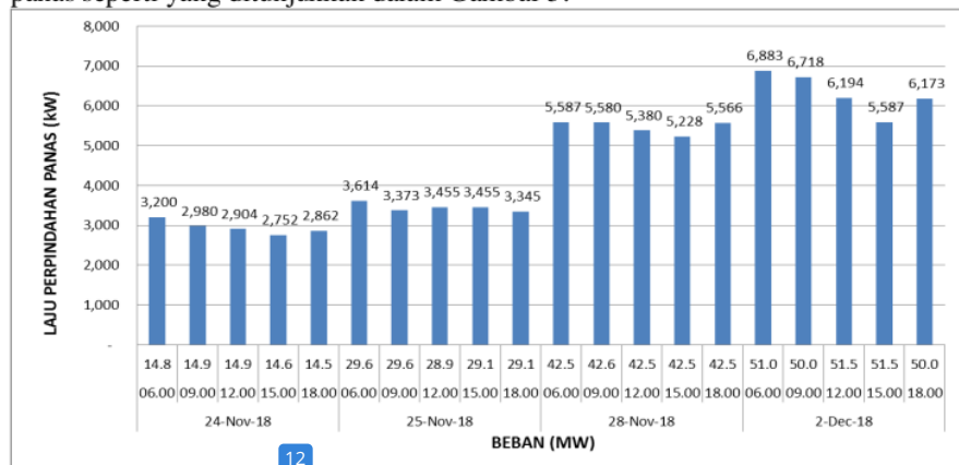
12 Gambar 5. Laju Perpindahan Panas
