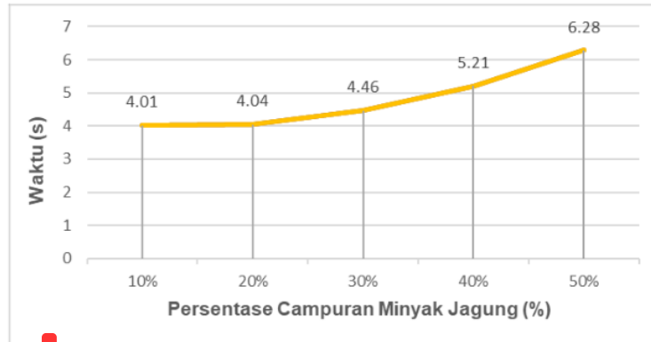
Gambar 3. Grafik pengaruh persentase campuran minyak jagung – solar terhadap ignition delay time
