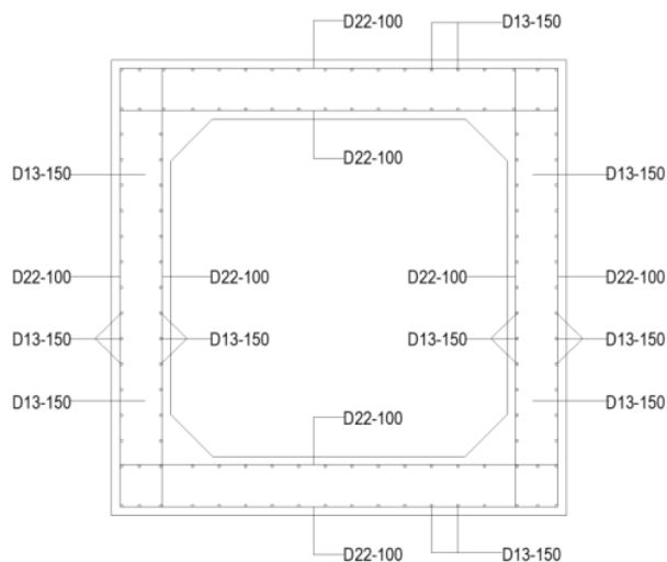
Gambar 8. Desain penulangan box culvert
