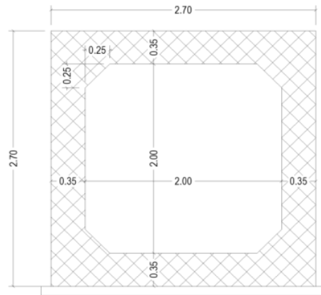
Gambar 4. Geometri Perencanaan Box Culvert
