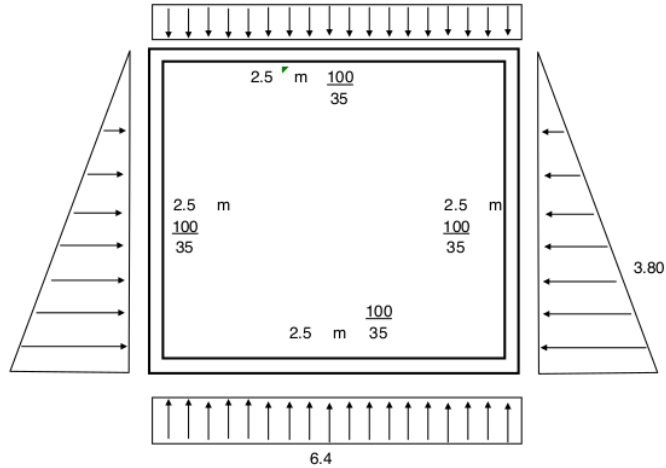
Gambar 5. Diagram Pembebanan pada Box Culvert
