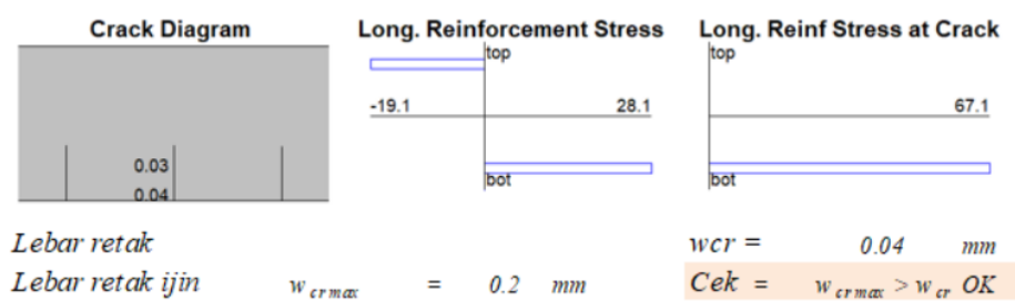
Gambar 7. Diagram Retak Penampang, Crack = 0,04 mm
