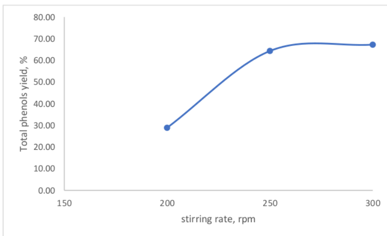
Gambar 2. Yield total fenol yang dihasilkan dari ekstraksi dengan kecepatan pengadukan yang berbeda.
