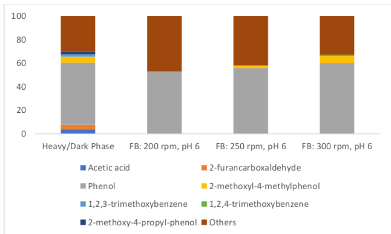
Gambar 1. Fase berat bio-oil (HBO) dan hasil ekstraksinya (FB) pada kecepatan pengadukan yang berbeda.
