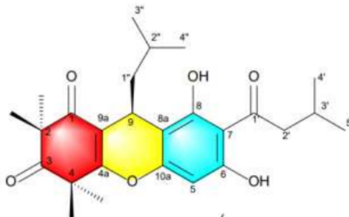
Gambar 8.1 Struktur dari rhodomyrtone (Zhao et al. , 2020)
