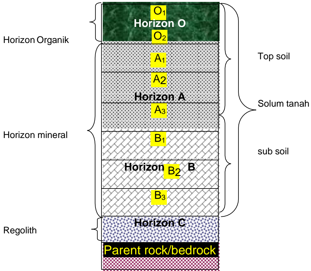
Gambar 5.1 Profil Tanah
