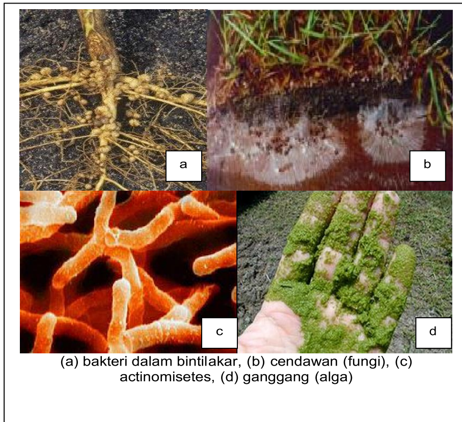
Gambar 7.14. Mikroflora Tanah
