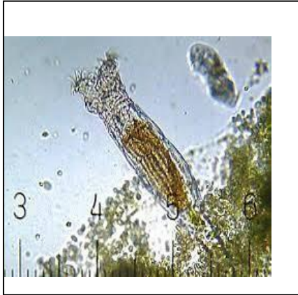
Gambar 7. 13. Rotifera
