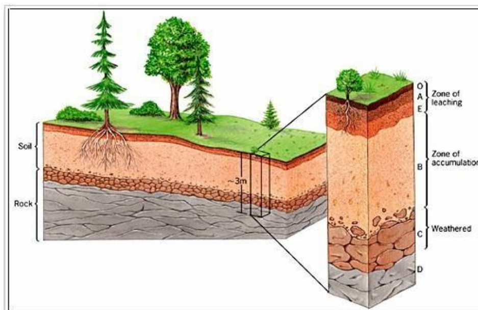
Gambar 2.1 Tubuh Tanah
