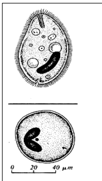
Gambar 7.11. Protozoa
