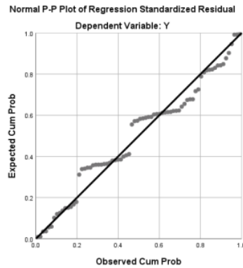
Gambar 2. Sebaran plot pada Uji Normalitas Data
