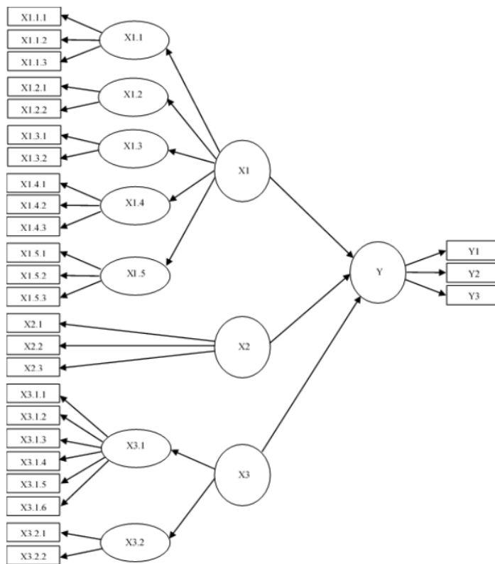
Gambar 1. Model struktural kerangka penelitian
