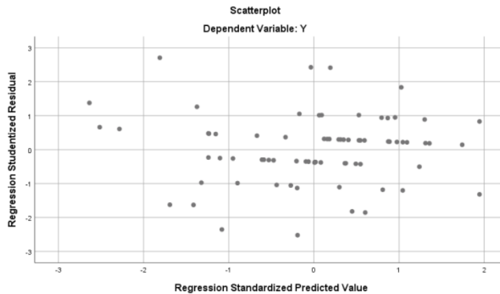
Gambar 3. Sebaran pola Scatter Plot
