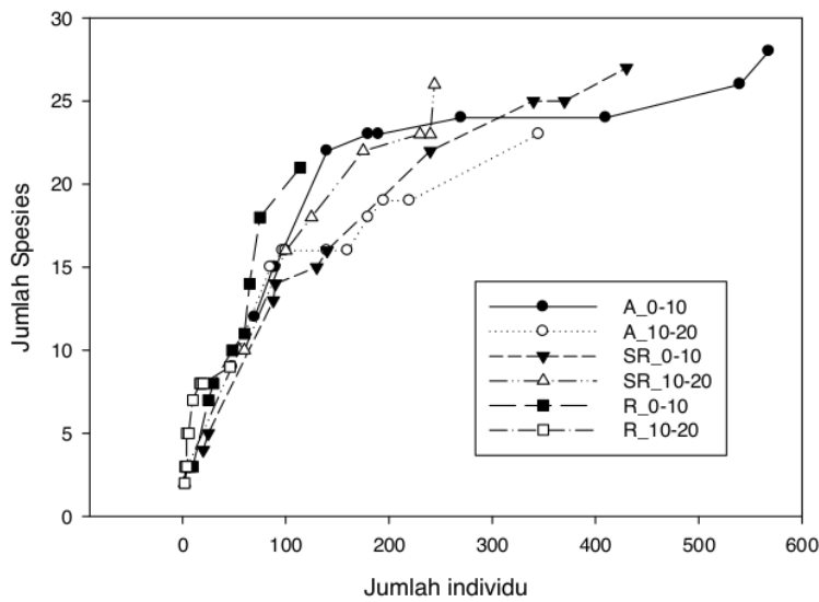
Gambar 1. Kurva akumulasi spesies berdasarkan-sampel (atas) dan berdasarkan-individu (bawah) untuk nematoda tanah di lahan bekas tambang batubara pada tiga lokasi dan dua kedalaman. A: alami; SR: setengah rusak; R: rusak. 0-10: kedalaman 0-10 cm; 10-20: kedalaman 10-20 cm.
