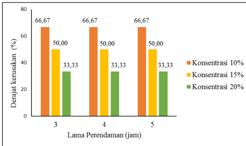
Gambar 5. Grafik nilai rata-rata derajat kerusakan kayu nangka (%)
