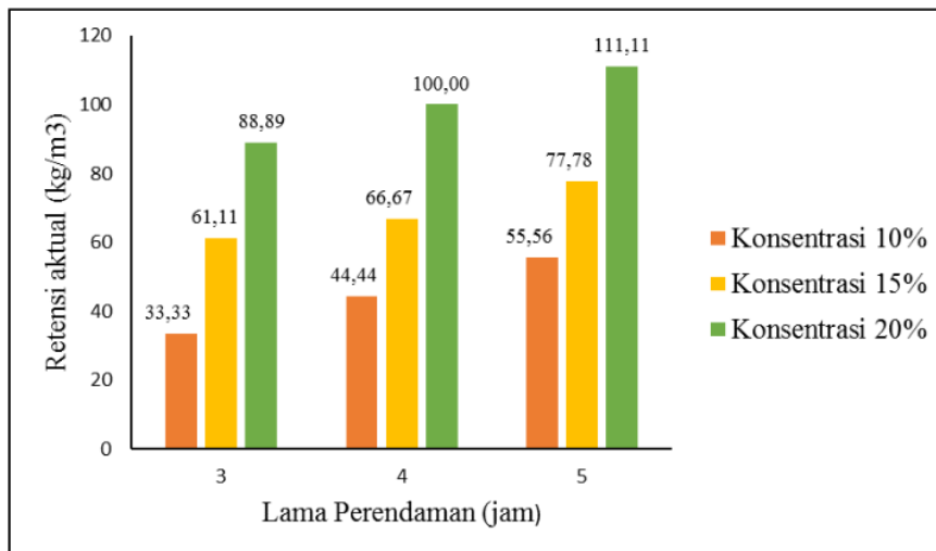
Gambar 3. Grafik rata-rata nilai retensi aktual (kg/m 3 )
