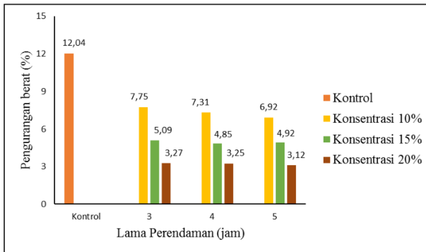
Gambar 4. Grafik nilai rata-rata pengurangan berat kayu nangka (%)
