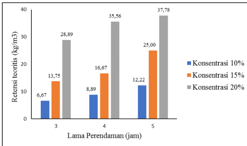
Gambar 2. Grafik rata-rata nilai retensi teoritis (kg/m 3 )
