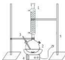
Gambar 1. Rangkaian Alat Hidrolisa
