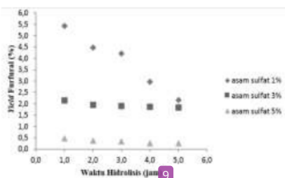
Gambar 3. Hubungan antara Konsentrasi Asam Sulfat dan Waktu Hidrolisis terhadap Perolehan Kadar Furfural.
