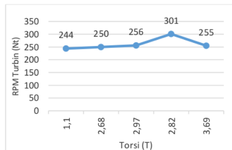
Gambar 8. Hubungan Antara Torsi dengan RPM terhadap Debit
