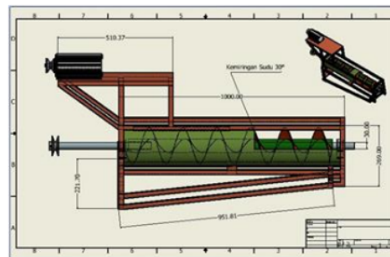
Gambar 3. Lembar Kerja Rancangan PLTPH
