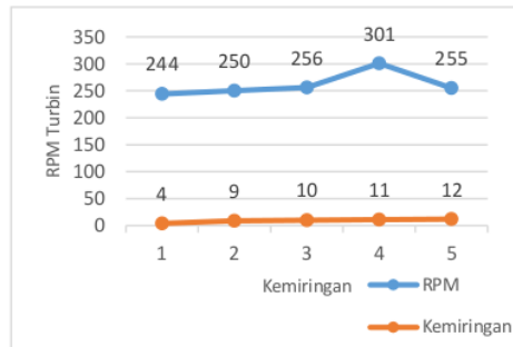
Gambar 9 Hubungan Antara Kemiringan Terhadap RPM
