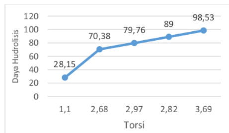
Gambar 9 Hubungan Antara Daya Hidrolisis Terhadap Torsi
