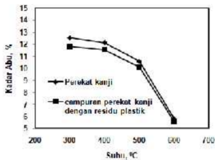
Gambar 5. Pengaruh Jenis Perekat Terhadap Kadar Abu
