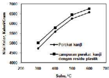
Gambar 3. Pengaruh Jenis Perekat Terhadap Nilai Kalor
