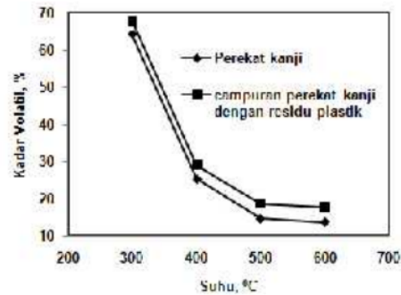
Gambar 6. Pengaruh Jenis Perekat Terhadap Kadar Volatil Kalor
