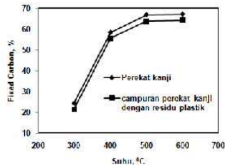
Gambar 7. Pengaruh Jenis Perekat Terhadap Fixed Carbon
