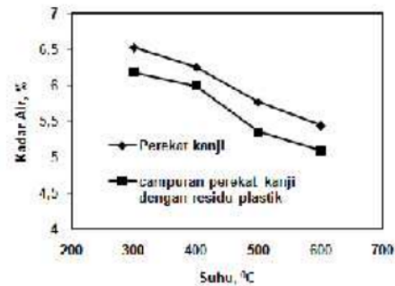
Gambar 4. Pengaruh Jenis Perekat Terhadap Kadar Air
