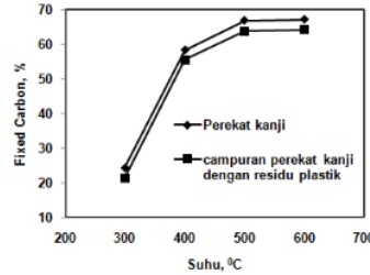
Gambar 6. Pengaruh Jenis Perekat Terhadap Fixed Carbon
