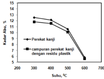
Gambar 4. Pengaruh Jenis Perekat Terhadap Kadar Abu
