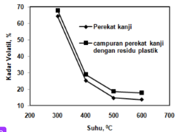
Gambar 5. Pengaruh Jenis Perekat Terhadap Kadar Volatil Kalor
