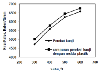
Gambar 2. Pengaruh Jenis Perekat Terhadap Nilai Kalor
