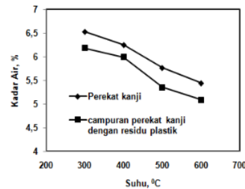
Gambar 3. Pengaruh Jenis Perekat Terhadap Kadar Air
