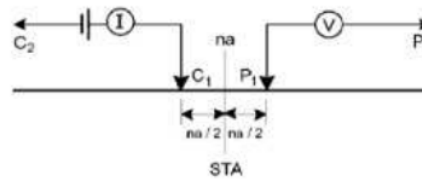
Gambar 1. Susunan elektroda konfigurasi pole-pole
