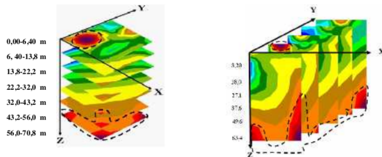
Gambar 4. Kontur resistivitas penampang horizontal dan vertikal
