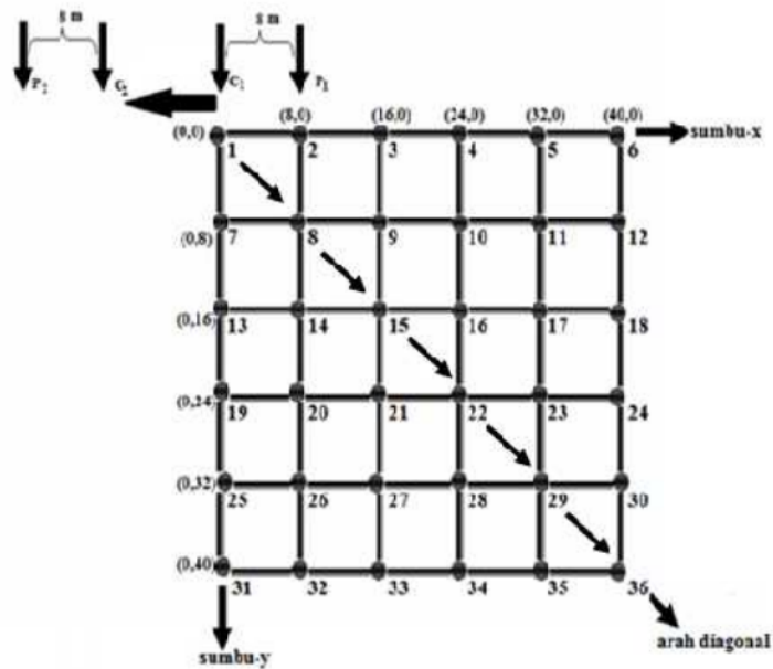
Gambar 3. Skema pengambilan data di lapangan
