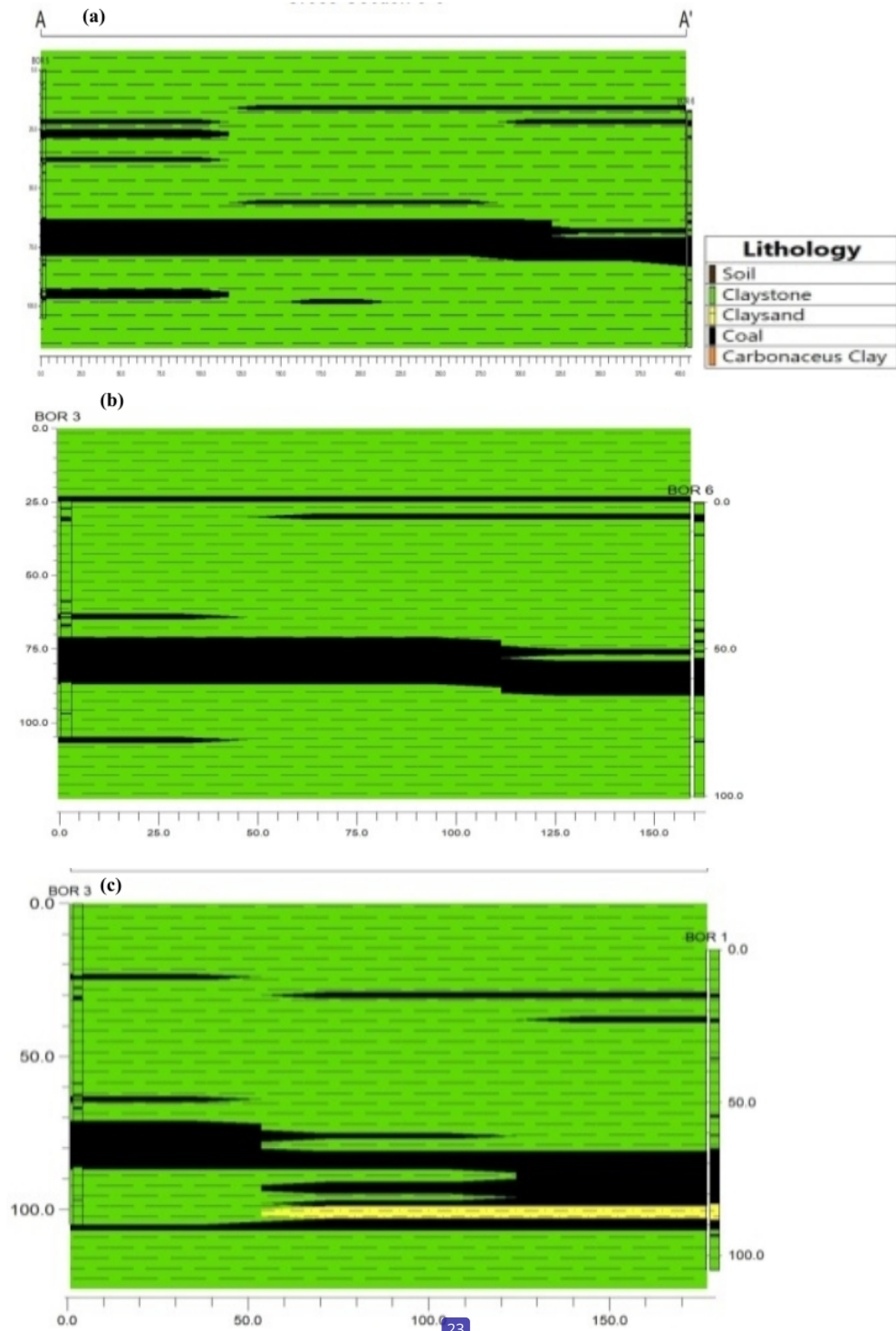
Gambar 6. Penampang melintang lintasan: (a) 5 dan 6, (b) 6 dan 3, dan (c) 3 dan 1
