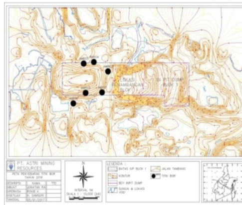
Gambar 2. Peta Sebaran Titik Bor
