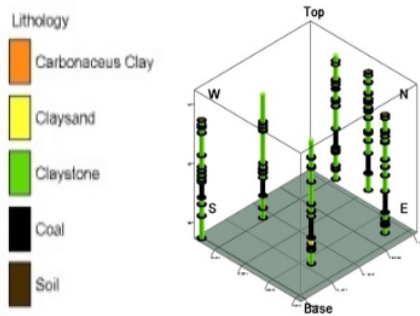
Gambar 9. Striplog sebaran batubara 3D
