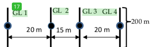
Gambar 4. Sketsa Pengambilan Data Lapangan
