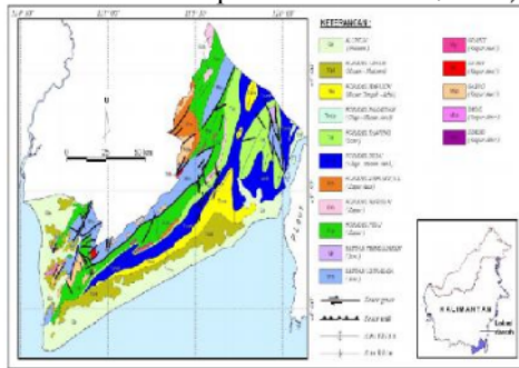
Gambar 1. Peta Geologi Kab. Tanah Laut
