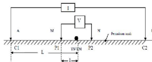
Gambar 2. Konfigurasi elektroda Schlumberger (Telford, 1990)
