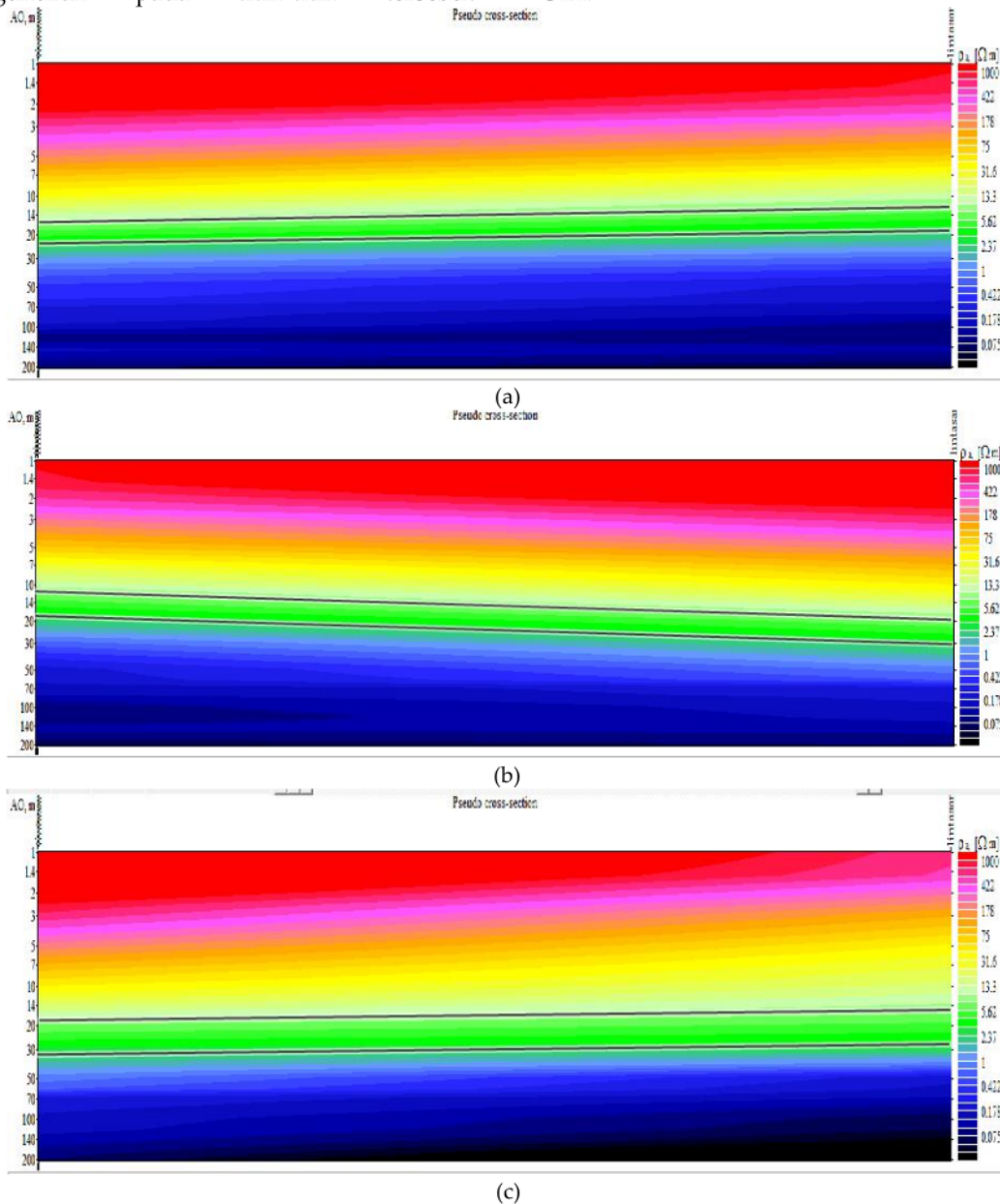
Gambar 5. Titik Sounding (a) GL 1 dan GL 2, (b) GL 2 dan GL 3, dan (c) GL 3 dan GL 4
