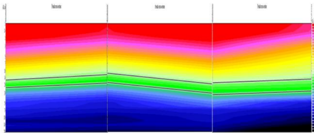
Gambar 6. Titik Sounding GL1, GL2, GL3, dan GL4
