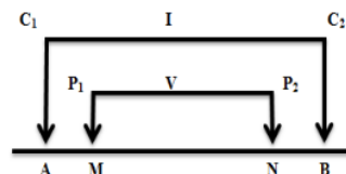
Gambar 1. Konfigurasi Schlumberger.
