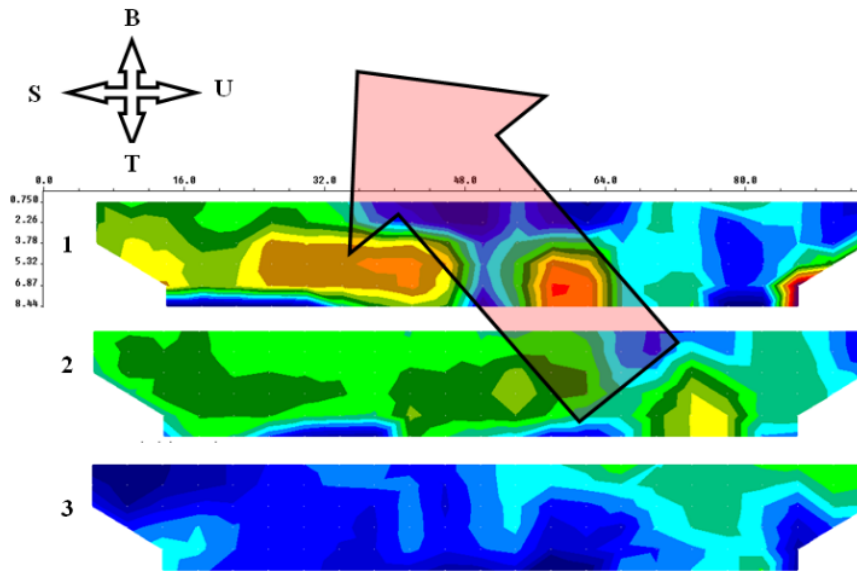
Gambar 4. Penampang resistivitas 2D disusun secara berurutan
