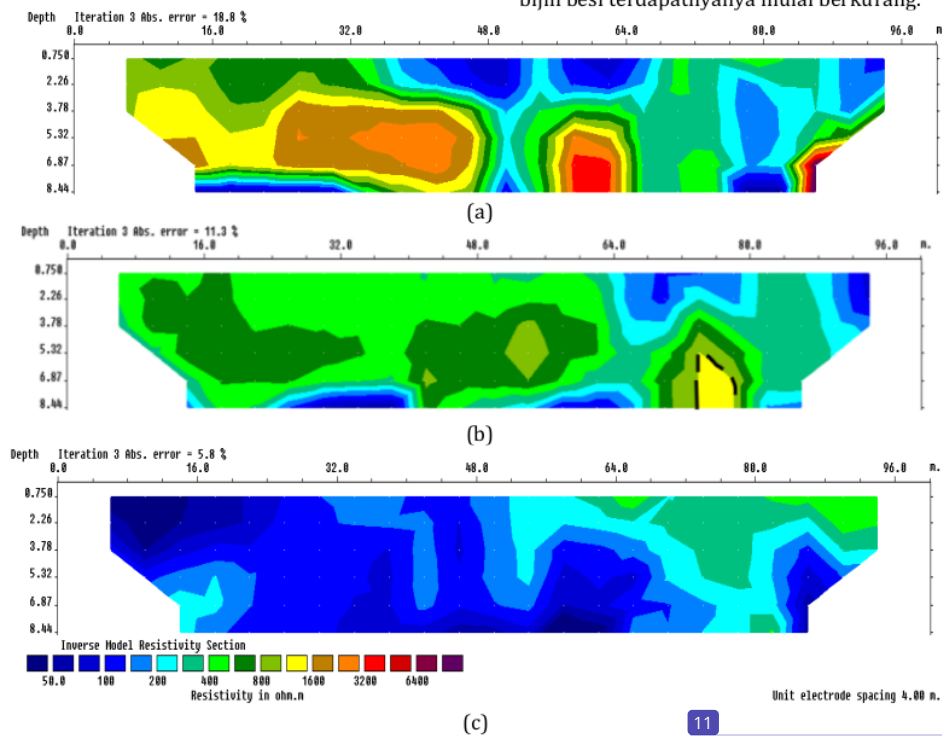
Gambar 3. Penampang resistivitas 2D hasil pengolahan res2dinv pada (a) lintasan 1, (b) lintasan 2, dan (c) lintasan 3
