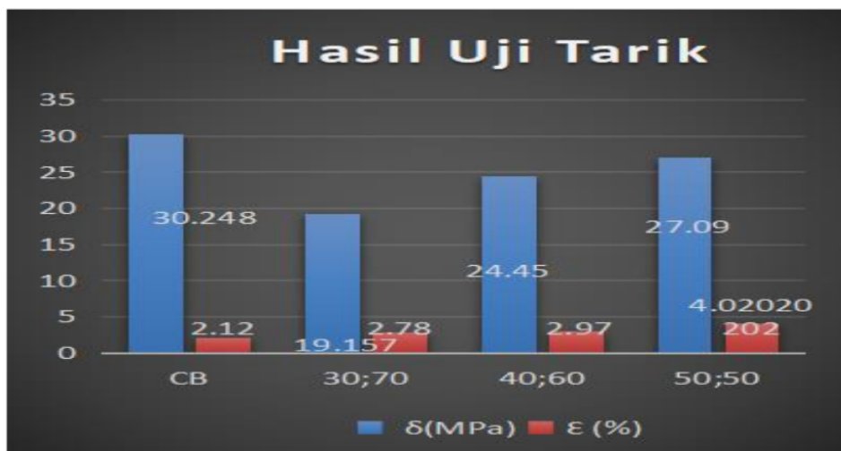
Gambar 2. Grafik Hasil Uji Tarik
