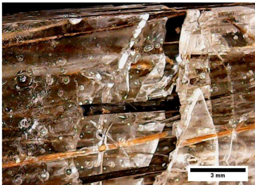
Gambar 5. Foto Mikro Patahan Spesimen Komposit Komposisi 40:60
