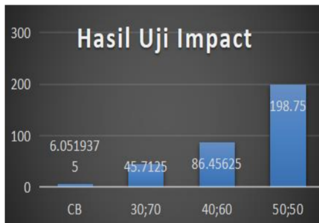
Gambar 1. Grafik Hasil Uji Impak
