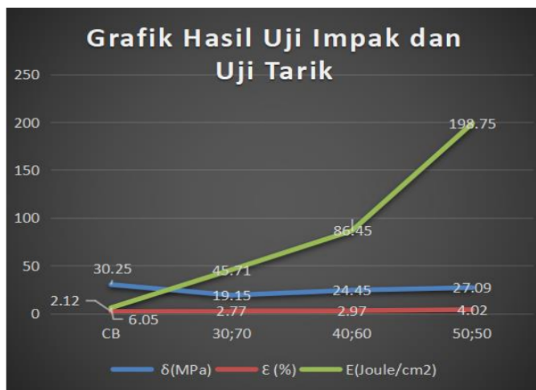
Gambar 3. Grafik Hasil Uji Impak dan Uji Tarik
