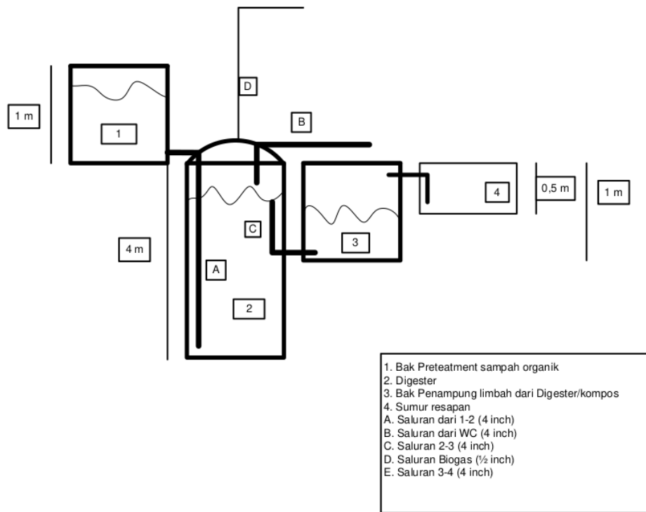
Gambar 1. Desain Teknologi Digester yang diterapkan
