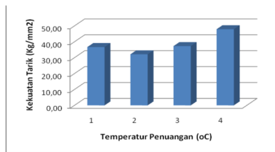
Gambar 4. Grafik hubungan temperatur penuangan dengan tegangan tarik
