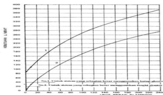
Gambar 1. Kurva Perkiraan Beban Kebutuhan Alat Plumbing
