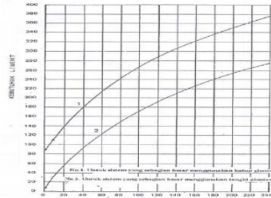
Gambar 3. Kurva perkiraan beban kebutuhan air untuk UBAP 240
