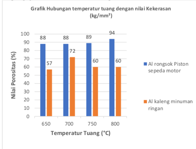
Gambar 4. Grafik Hasil Uji Kekerasan Vickers
