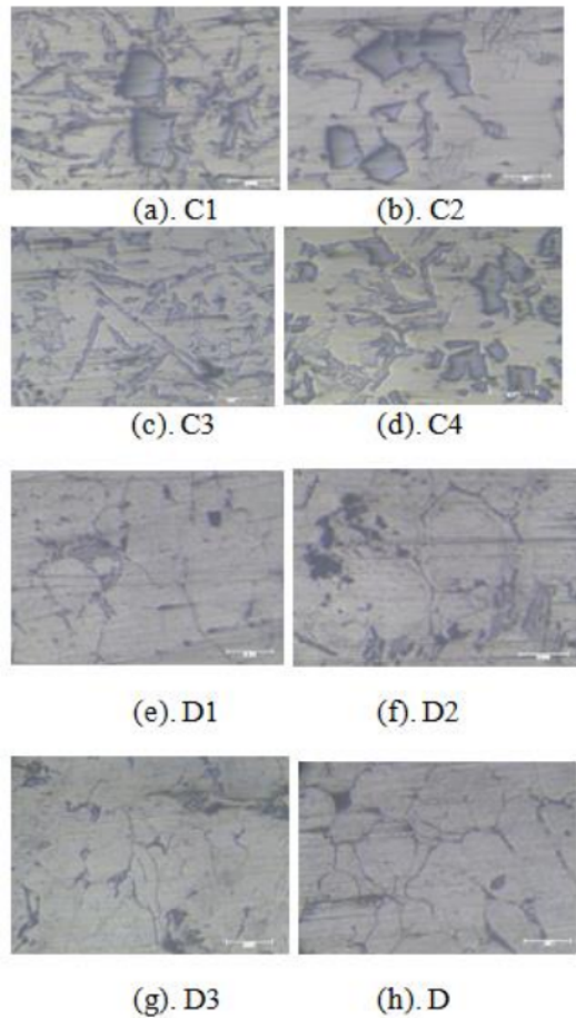
Gambar 2. Foto Hasil Struktur Mikro Dengan Perbesaran 101 X
