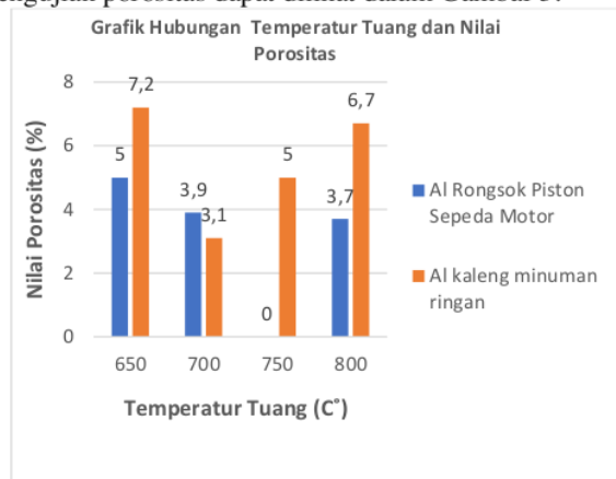
Gambar 3. Grafik Hasil Uji Porositas
