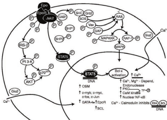
Gambar 7 Jalur transduksi sinyal EpoR-JAK2/STAT5/Bcl-x 41
