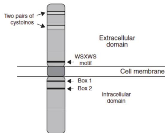
Gambar 4 Skema struktur reseptor eritropoetin 32
