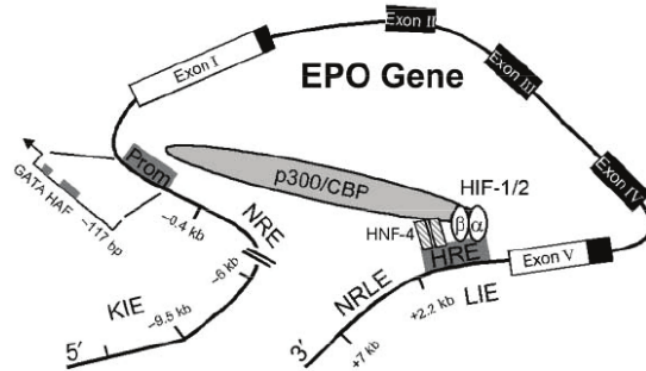
Gambar 1 Regulasi gen eritropoetin (EPO) yang tergantung oksigen 20
