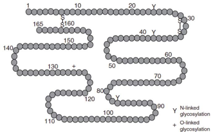
Gambar 2 Struktur eritropoetin 10
