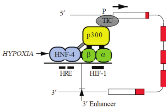
Gambar 3 Model perakitan faktor-faktor transkripsi di regio 3' enhancer gen Epo untuk mengaktivasi transkripsi gen Epo 3
