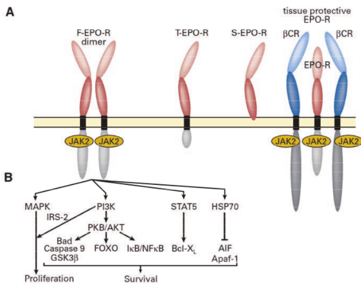
Gambar 5 Pensinyalan eritropoetin (Epo) dan Epo reseptor (EpoR) 35
