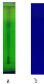
Gambar 2. Kromatogram KLT ekstrak akar pedada di bawah lampu UV 254 (a) dan UV 366 (b)
