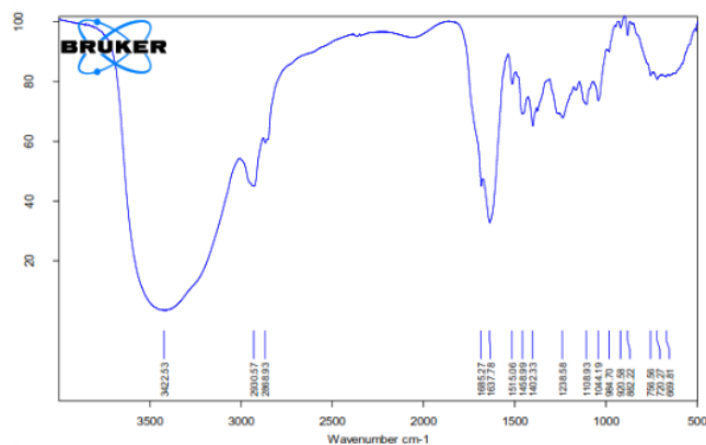
Gambar 3. Spektra infra merah ekstrak akar pedada
