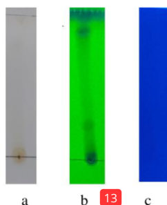
Gambar 1. Kromatogram KLT ekstrak akar di bawah sinar tampak (a), sinar UV 254 (b), sinar UV 366 (c)
