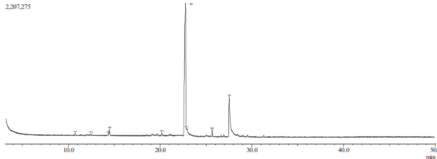
Gambar 1. Kromatogram GC minyak kayu manis asal Loksado
