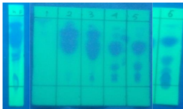
Gambar 2. Kromatogram KLT hasil fraksinasi minyak kayu manis
