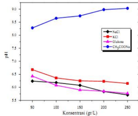
Gambar 3. Grafik hubungan konsentrasi osmotic agent dengan pH
