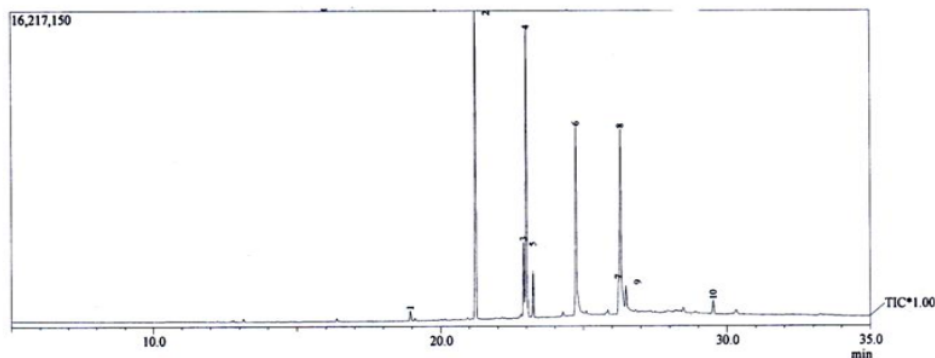
Gambar 6. Kromatogram GC metil ester Synechococcus sp
