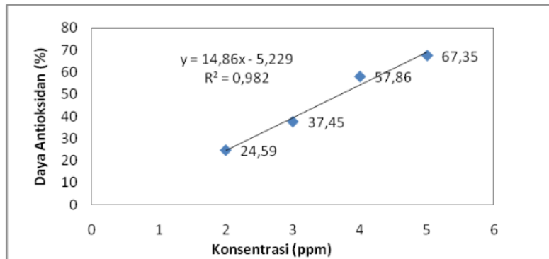
Gambar 1. Grafik Hubungan Konsentrasi dengan Daya Antioksidan Senyawa
