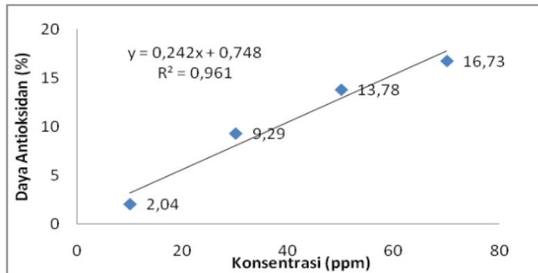
Gambar 1. Grafik Hubungan Konsentrasi dengan Daya Antioksidan Senyawa
