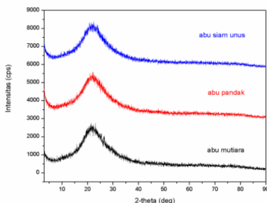
Gambar 11. Pola difraksi sinar-X pada masing-masing abu sekam
