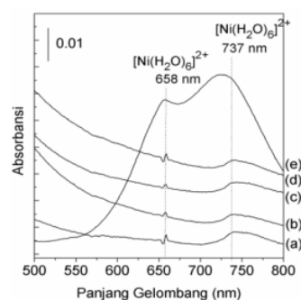
Gambar 1. Spektra UV-Vis larutan kompleks Ni 2+ dan supernatan setelah proses hidrotermal dengan rasio mol Ni/Ag yang berbeda (a) 0,75; (b) 1,5; (c) 2,0; (d) 3,0; dan (e) [Ni(H 2 O) 6 ] 2+ standar.
